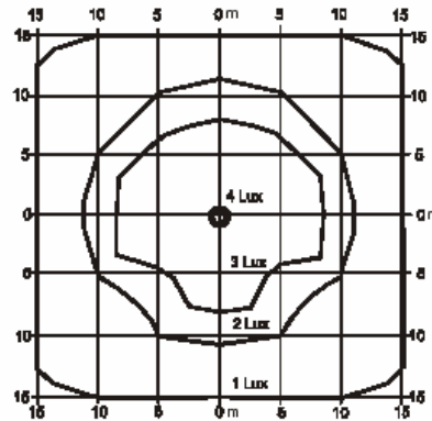
Leuchtcharakteristik aus 4m Lichtpunkthöhe
